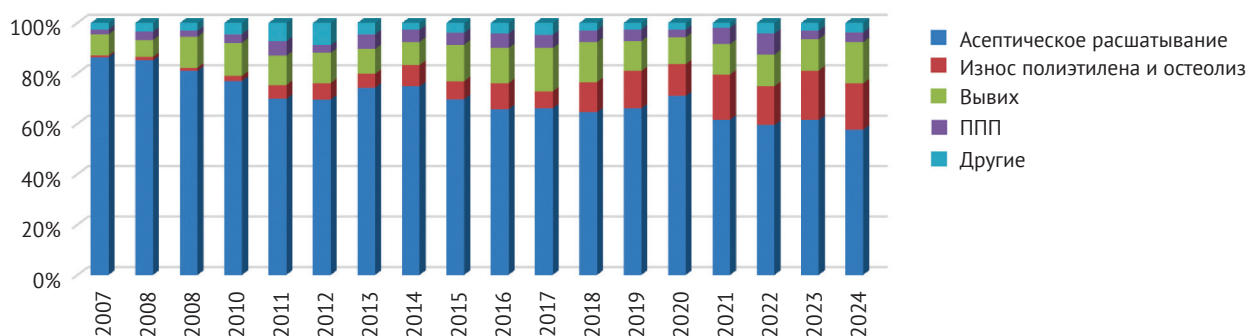
Рис. 10. Тенденции в изменении структуры причин асептической ревизии по годам Figure 10. Trends in the structure of aseptic revision causes by year
