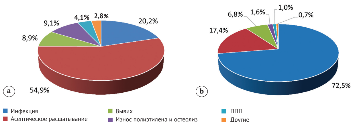
Рис. 9. Удельный вес различных причин ревизий: а — после первичного ЭП ТБС; б — после повторных ревизий Figure 9. Proportion of different causes of revision: а — after primary THA; б — after re-revisions
